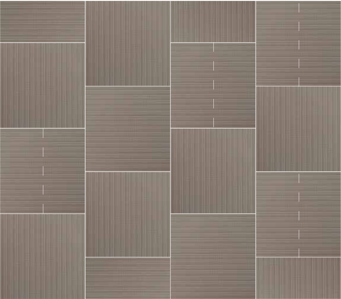
Patrón de instalación en escalera. Instalación sin juntas hasta 600 m² (30x20 m, con núcleo Hydrowood) Padrão de instalação da escada. Instalação sem juntas até 600 m² (30x20 m, com núcleo Hydrowood)
